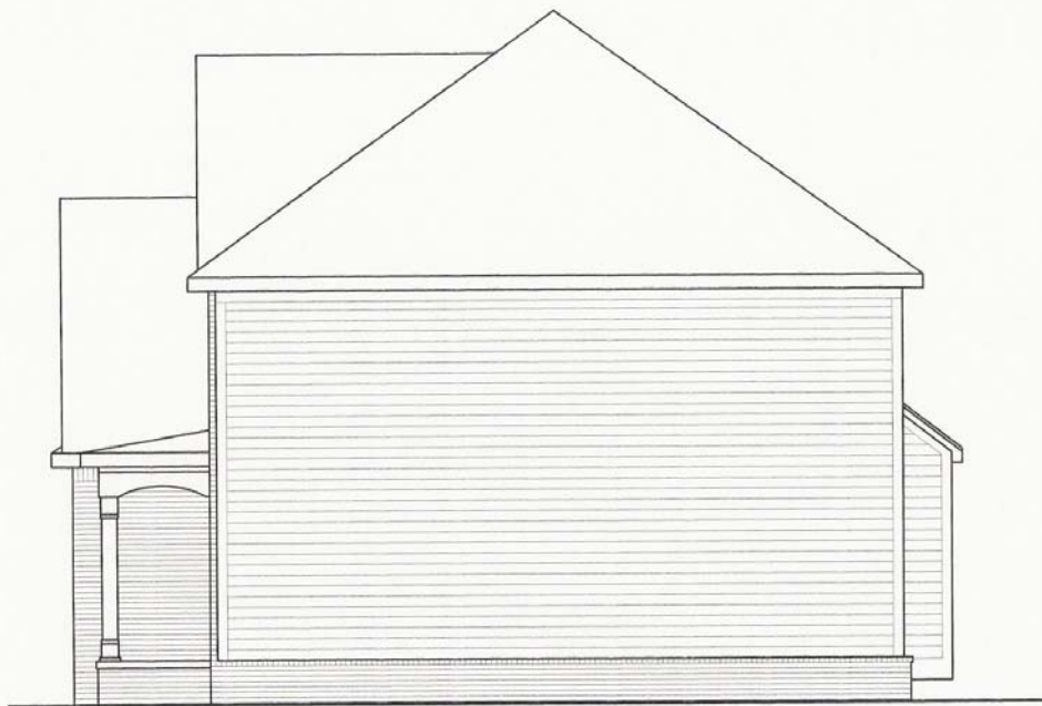
RIGHT ELEVATION
